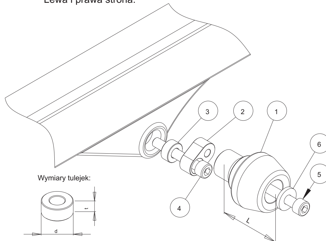
Schemat montażowy ślizgacza. Lewa i prawa strona.
