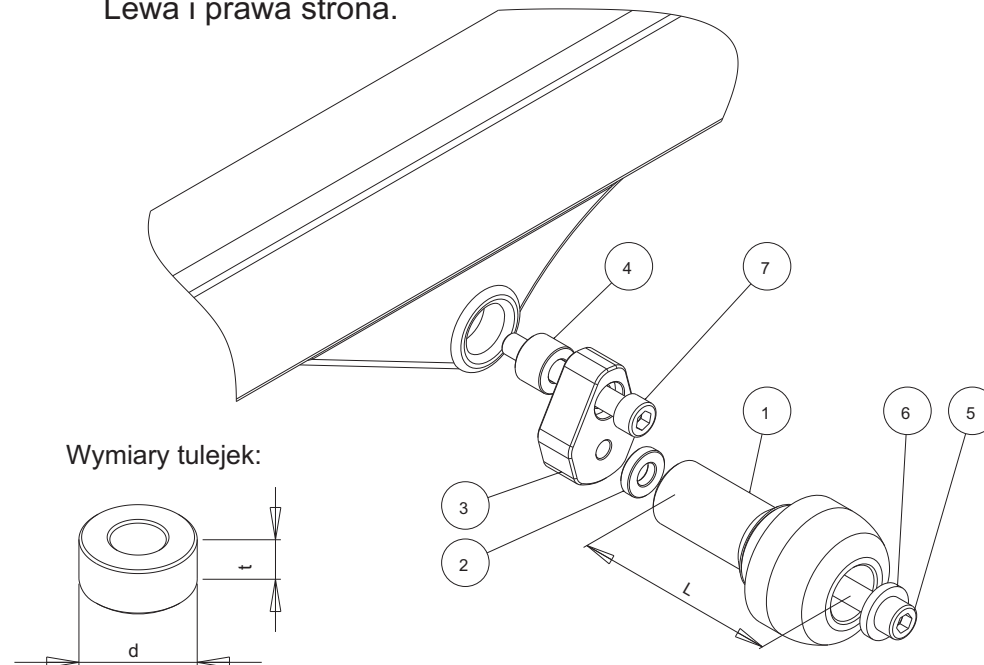
Schemat montażowy ślizgacza. Lewa i prawa strona.
