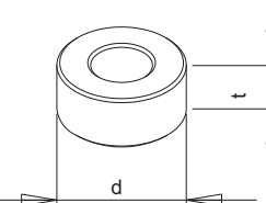
Wymiary tulejek:
