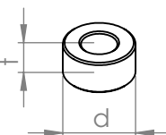
Wymiary tulejek
